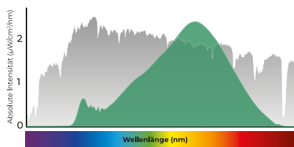
Das naturnahe Lichtspektrum der PureZ-NEO-LED Grauer Graph: Spektrum des natürlichen Tageslichts Grüner Graph: Typ. Spektrum der PureZ-Retro-LED
